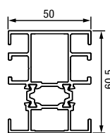
Rozširovací profil 50 mm
