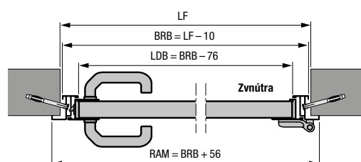
Vedľajšie dvere s hliníkovou rohovoú zárubňou typ profilu 1 alebo 2 Vnútroúny doraz
